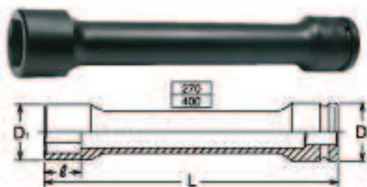
Douilles extra-longues pour écrous de roues
