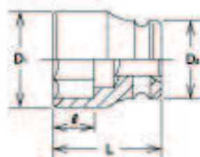
1840M Douilles 6 pans
