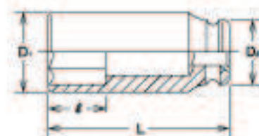
18400M Douilles 6 pans longues
